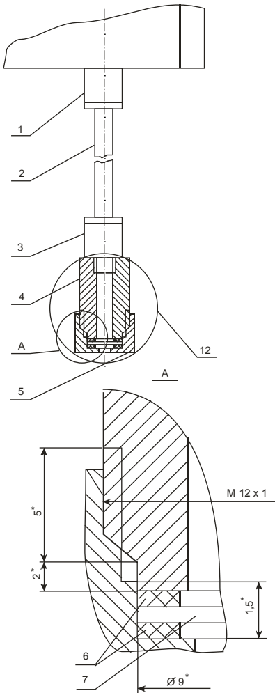
Пробоотборное устройство (вариант 1 и 2)
