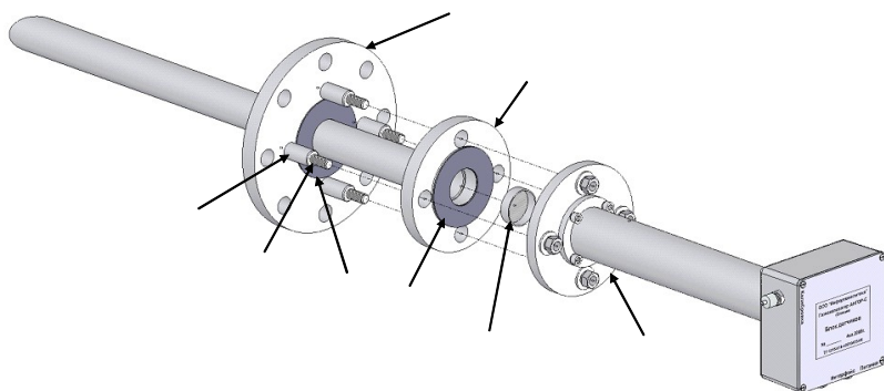
Рисунок 4 - Схема сборки блока датчиков
