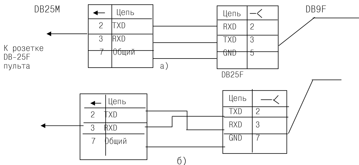
Рисунок 2.1 – Схема подключения пульта:
